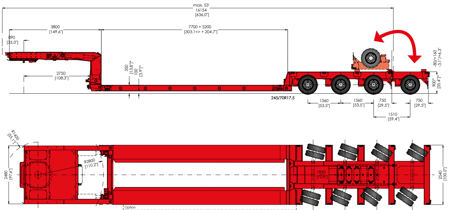
Mega-Z-3L-V-KBX-A-(US)Dock
